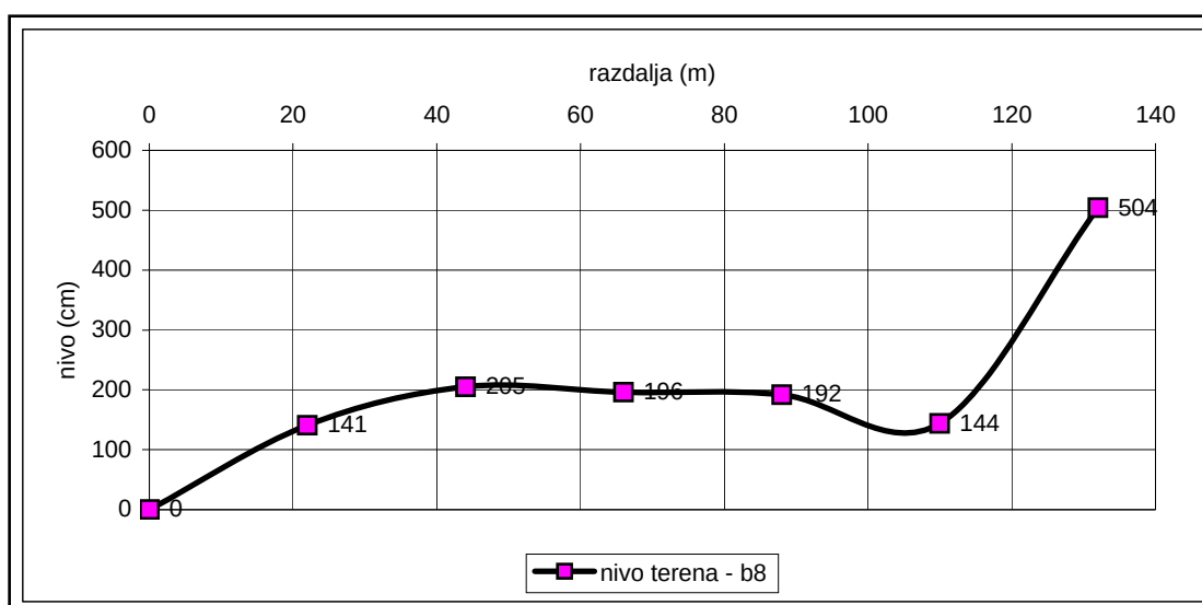
Grafikon 4: Prečni profil transekt na barju b8
