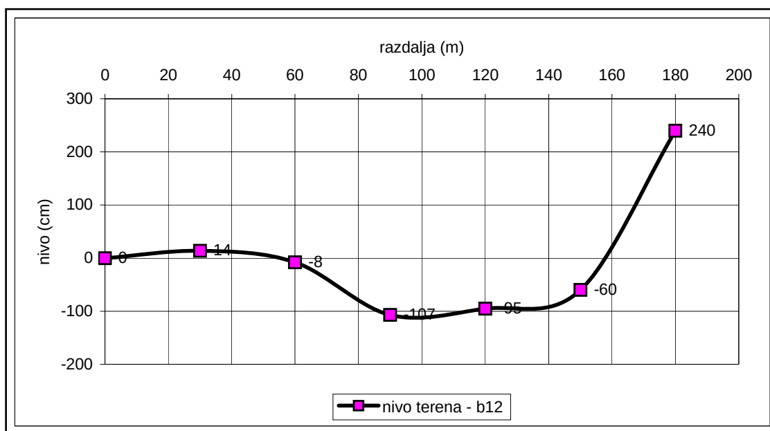
Grafikon 5: Prečni profil transeкта na barju b12
