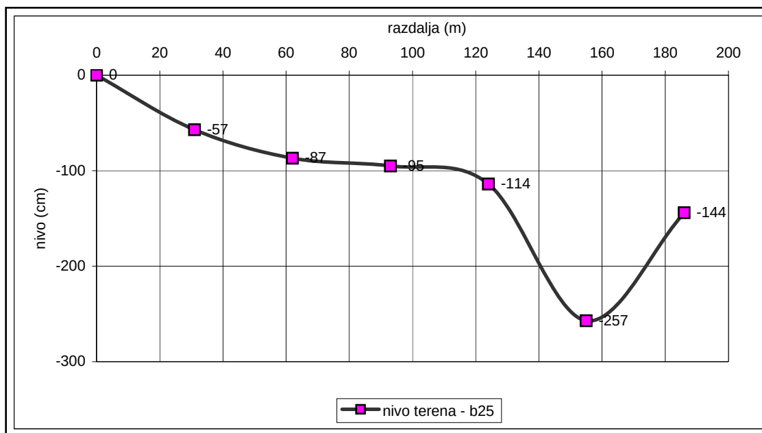
Grafikon 3: Prečni profil transeкта na barju b25
