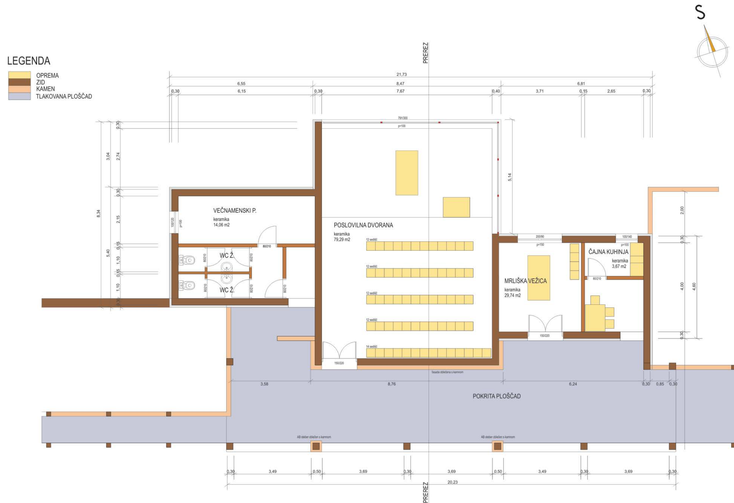
Slika 58: Nov pokopališki objekt – tloris 1:100
