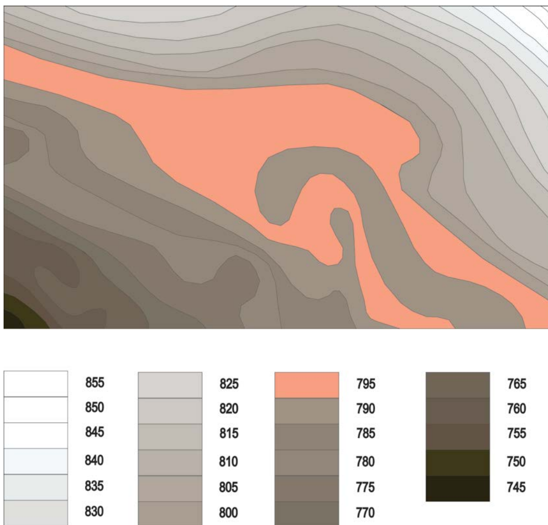
Slika 12: Višinski prikaz obravnavanega območja
