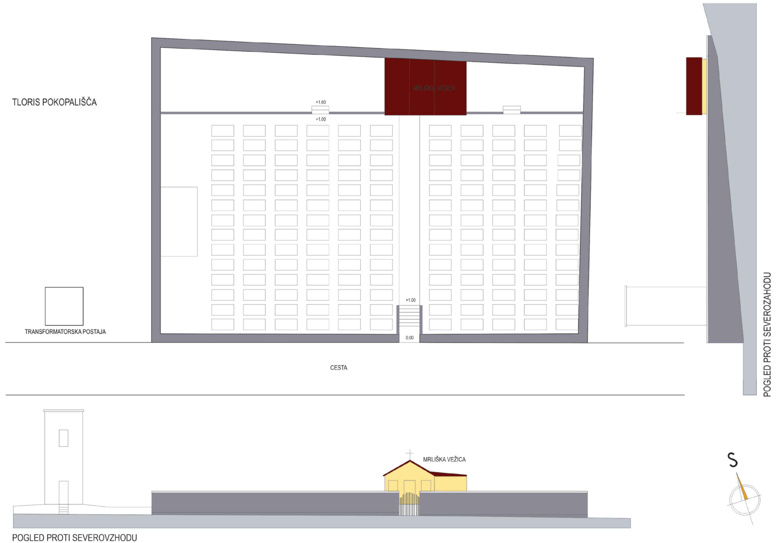
Slika 50: Tloris obstoječega pokopališča in pogledi 1:200
