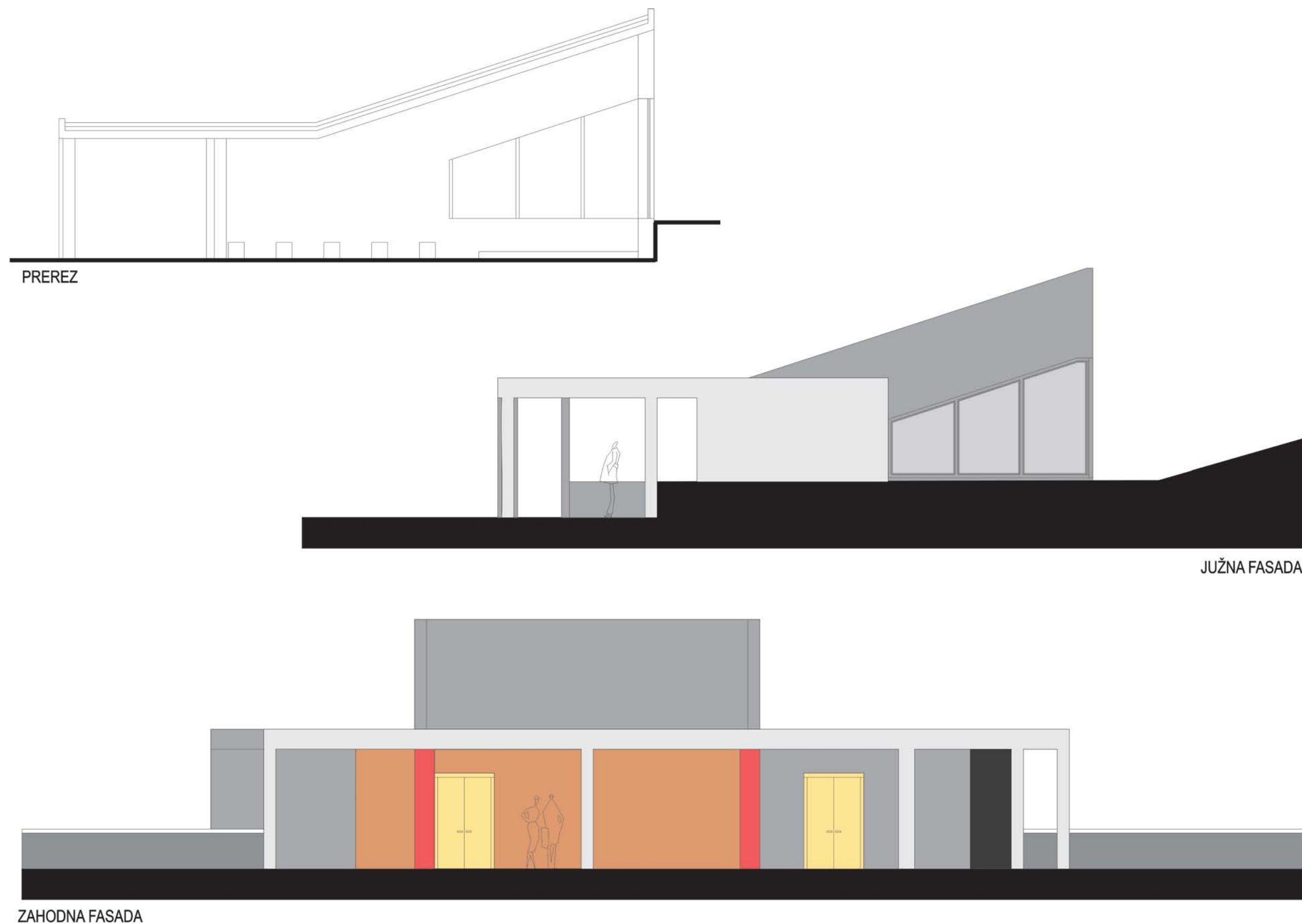
Slika 59: Nov pokopališki objekt- prerez in fasade 1:100
