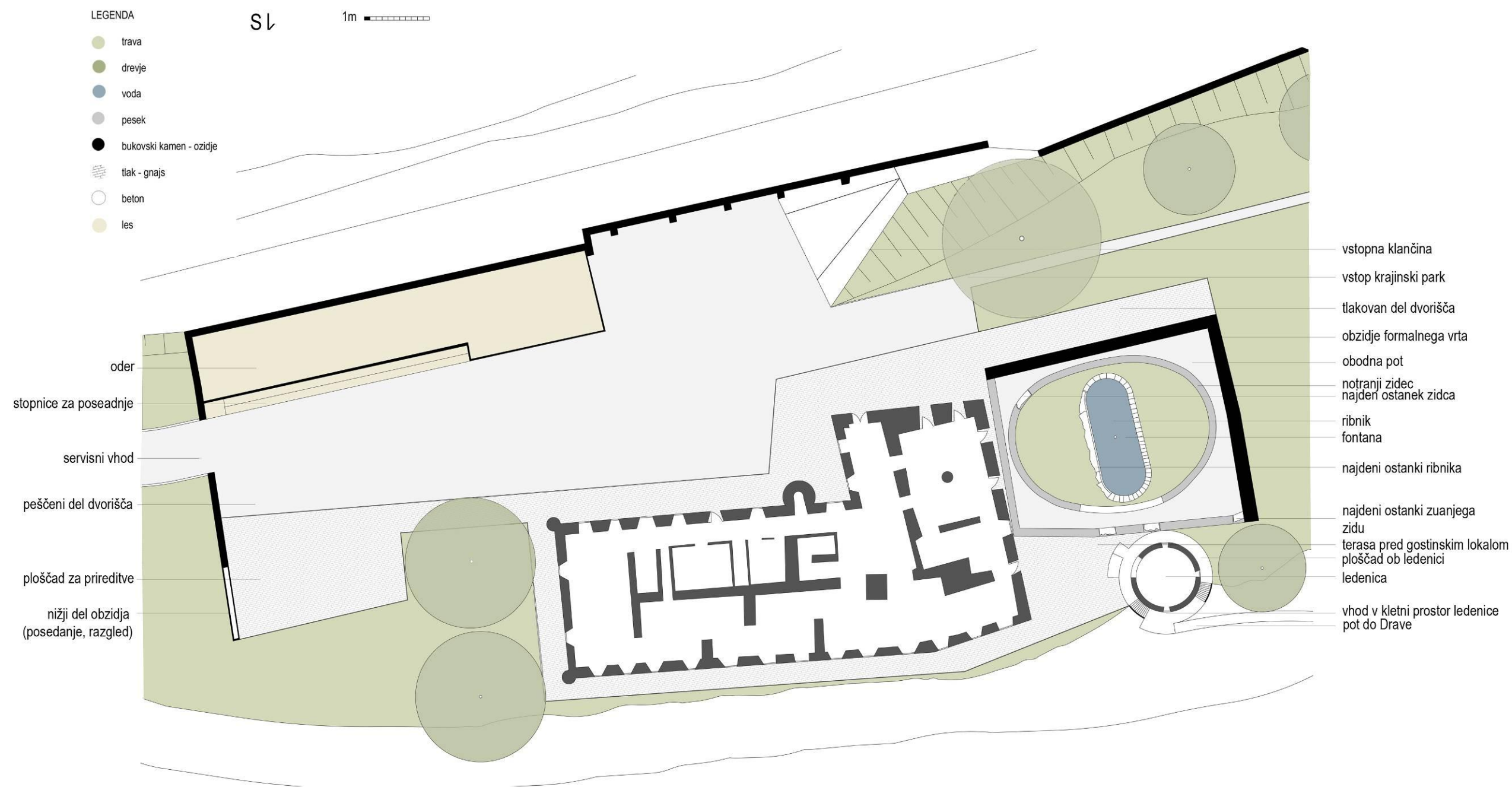
Slika 104: Predlog ureditve formalnega vrta in dvorišča ob dvorcu Bukovje
