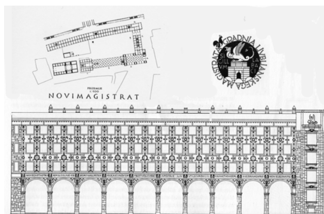
Slika 109: Izris novega magistrata (Krečič, 1992: 247)
