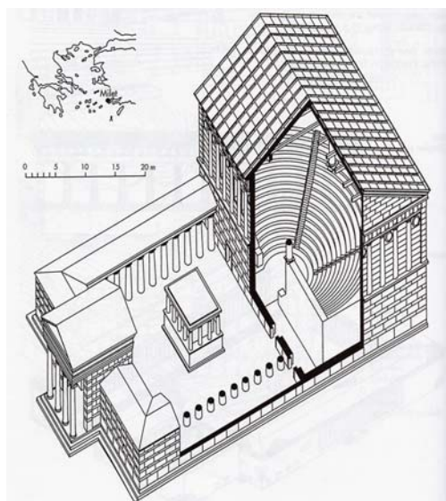
Slika 158: Bulevterij (175-164 pr. n. št.), Milet (Marinko, 1997: 210)
