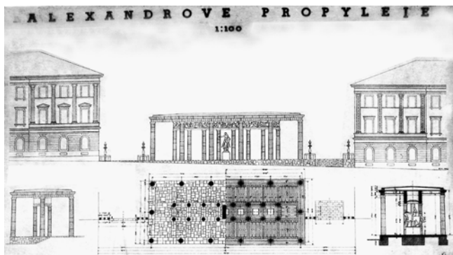
Slika 99: Aleksandrove propileje (Tepina, 1936)
